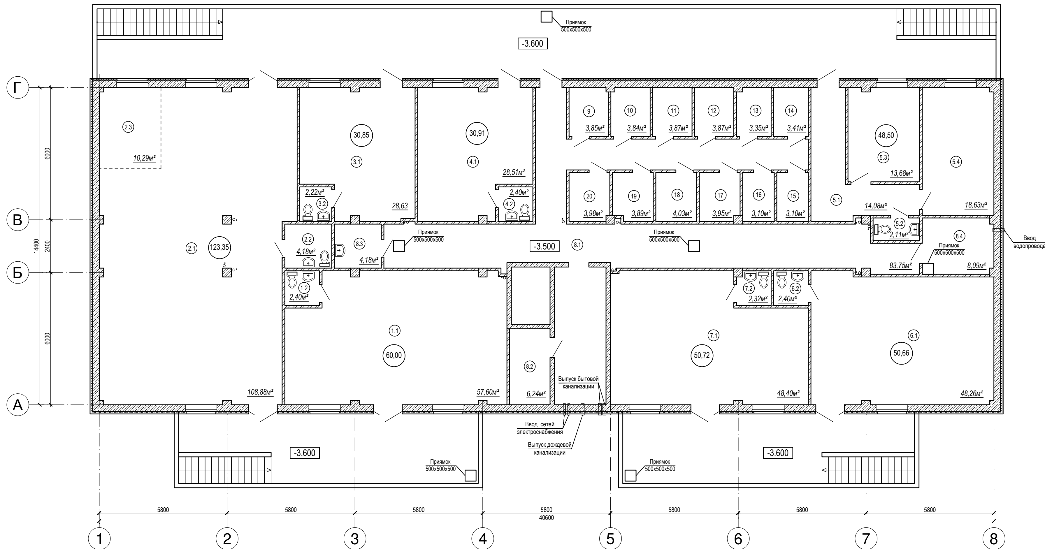
Экспликация помещений
